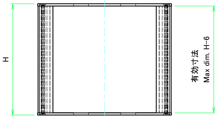
Wパネル1 / W Panel 1
